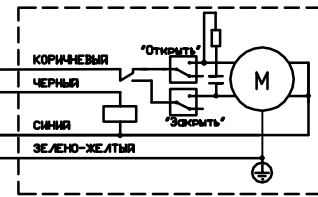
Шаровой электропривод "Gidrolock".
