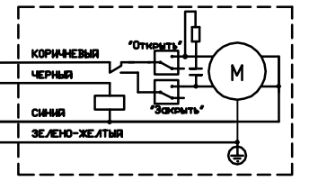
Шаровой электропривод "Gidrolock".
