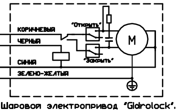
Шаровой электропривод "Gidrolock".
